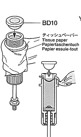
リヤダンパー (ロング)
