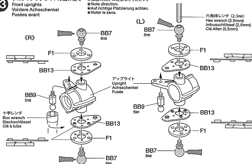
BB9 x2 5mmビローボール (長) Ball connector (long) Kugelkopf (lang) Connecteur à rotule (long)
