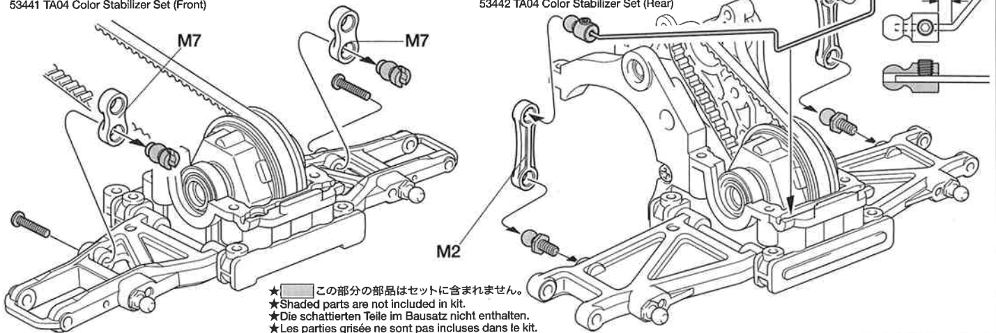
OP.442 TA04カラースタビライザーセット (リア) 53442 TA04 Color Stabilizer Set (Rear)
