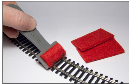
Schienenreiniger 15.PTC-001 Für Gleise Z, N, H0, 00
