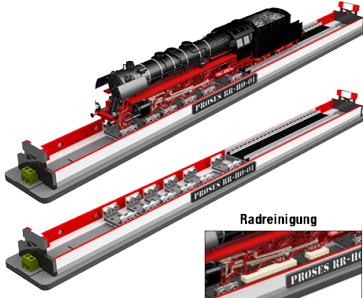
Rollenprüfstand 15.PRR-H0-01 H0 mit Radreinigungsfunktion
