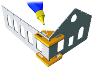
Rechtwinkel 15.PPR-SS-02 2 magnetische Halterungen mit 8 Festhaltemagneten
