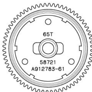
GB4 65T スパーギヤ ×1 65T Spur gear 65Z Hauptzahnrad Couronne 65 dents
