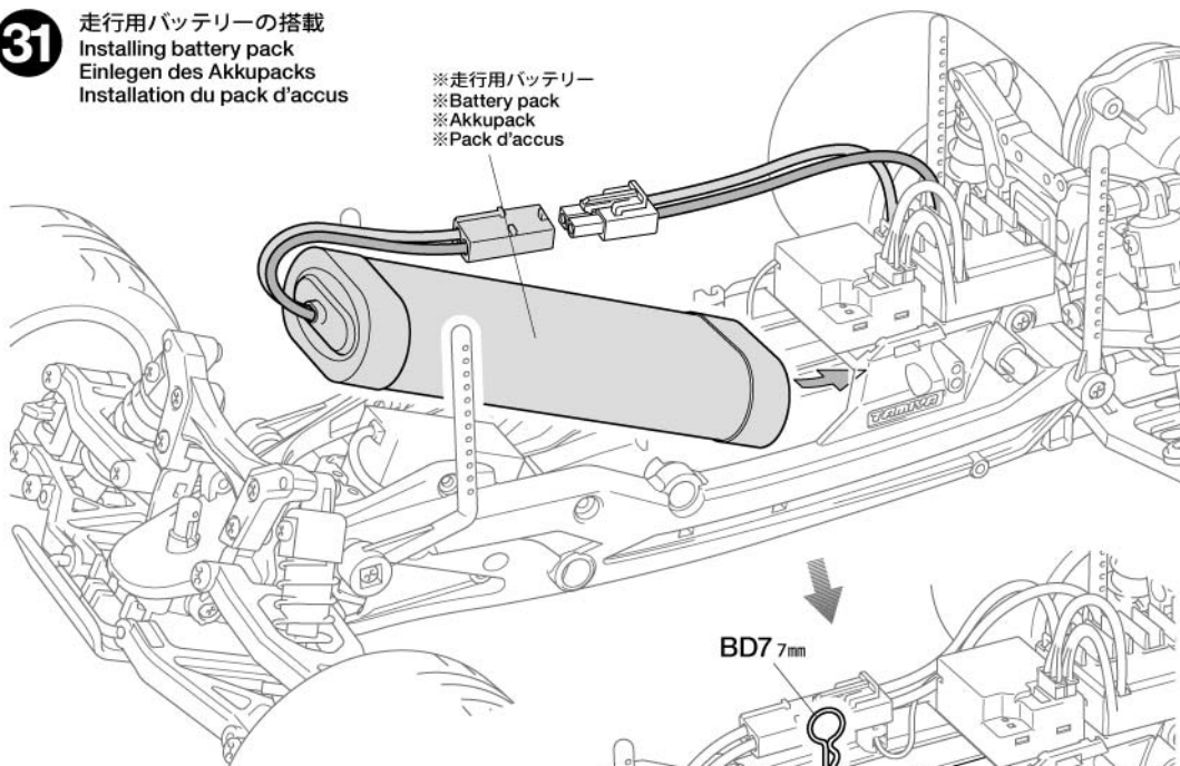
BD7 7mm スナップピン X1 Snap pin Federstecker Epingle métallique
